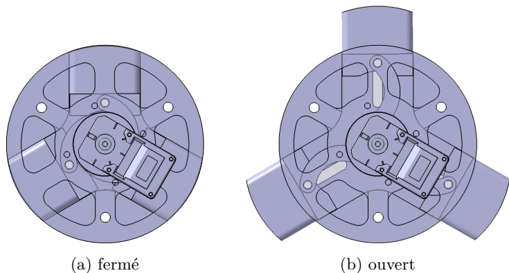
FIGURE 4.9 – Position des aérofreins d'SP-02
